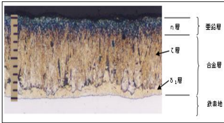
図-4 溶融亜鉛めっき被膜断面
